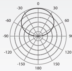
GSM Band H-Plane
