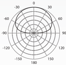
GSM Band H-Plane
